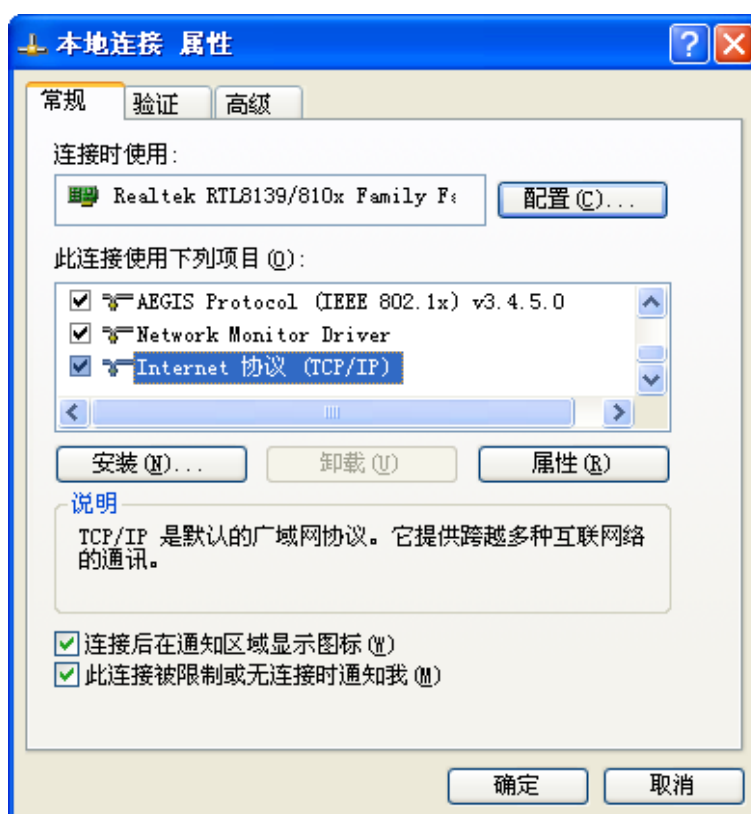
图 4 TCP/IP 协议属性
